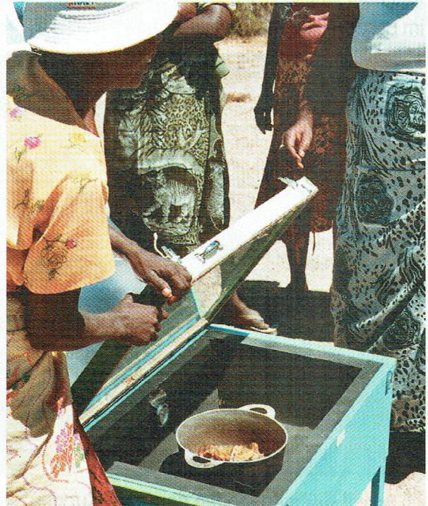
Madagaskar: Solarkocher im Einsatz Foto: ADES
